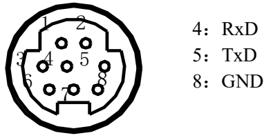
Mini Din 8 芯插座 (孔)
