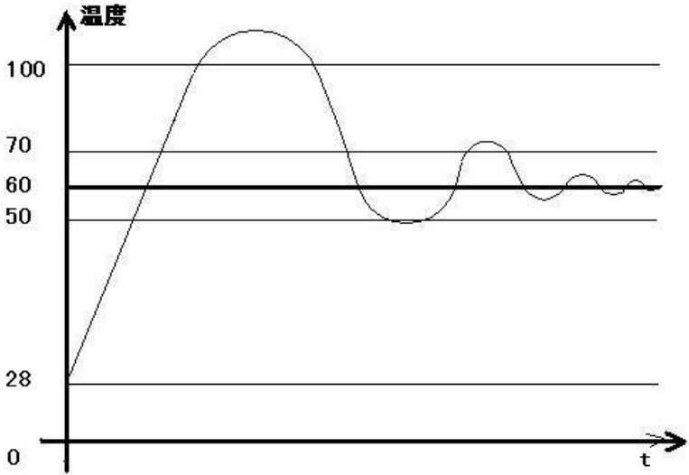
图 2 PID 自整定允许超调波形图
