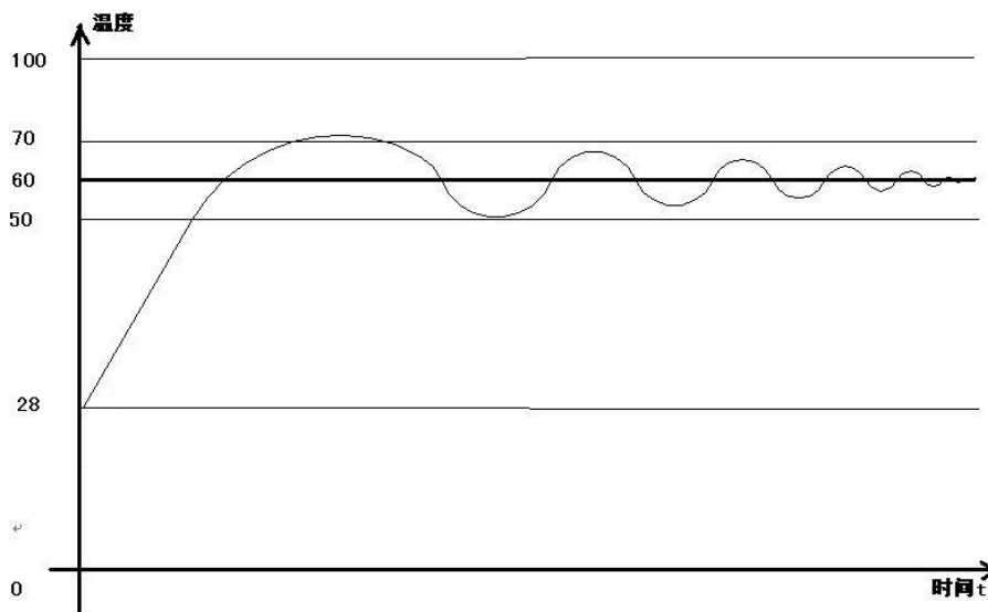
图 4 PID 自整定不允许超调波形图
