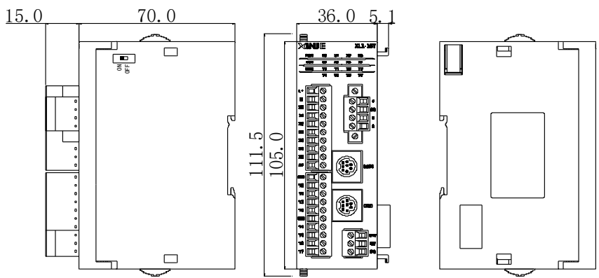
2-2-2. XL 系列外形尺寸图
