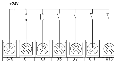
开关按钮接线图示例
