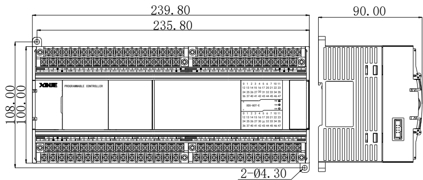
2-2-2. XL 系列外形尺寸图
