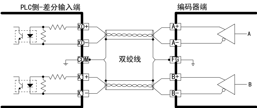
与编码器接线图示例
