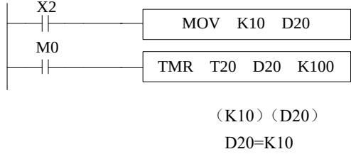
《定时器设定值的间接指定示例》
